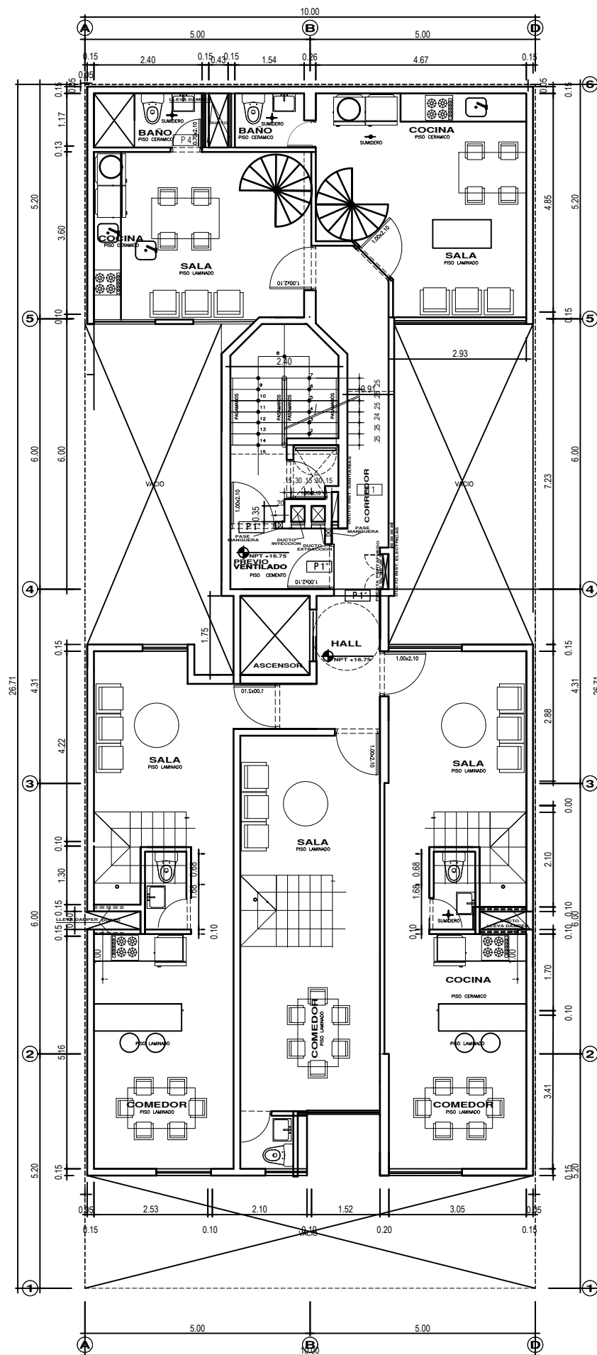
PLANTA 7mo piso
