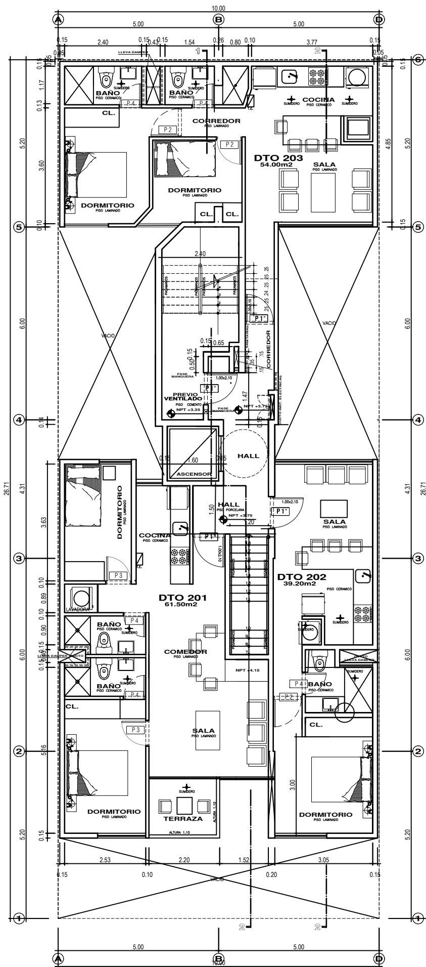
PLANTA SEGUNDO PISO
